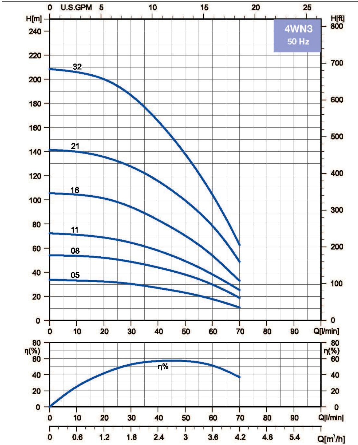
4WN3 – MEI > 0.70
