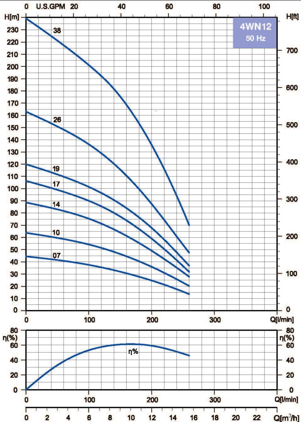
4WN12 – MEI > 0.10
