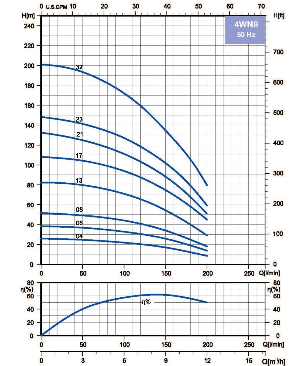
4WN8 – MEI > 0.10
