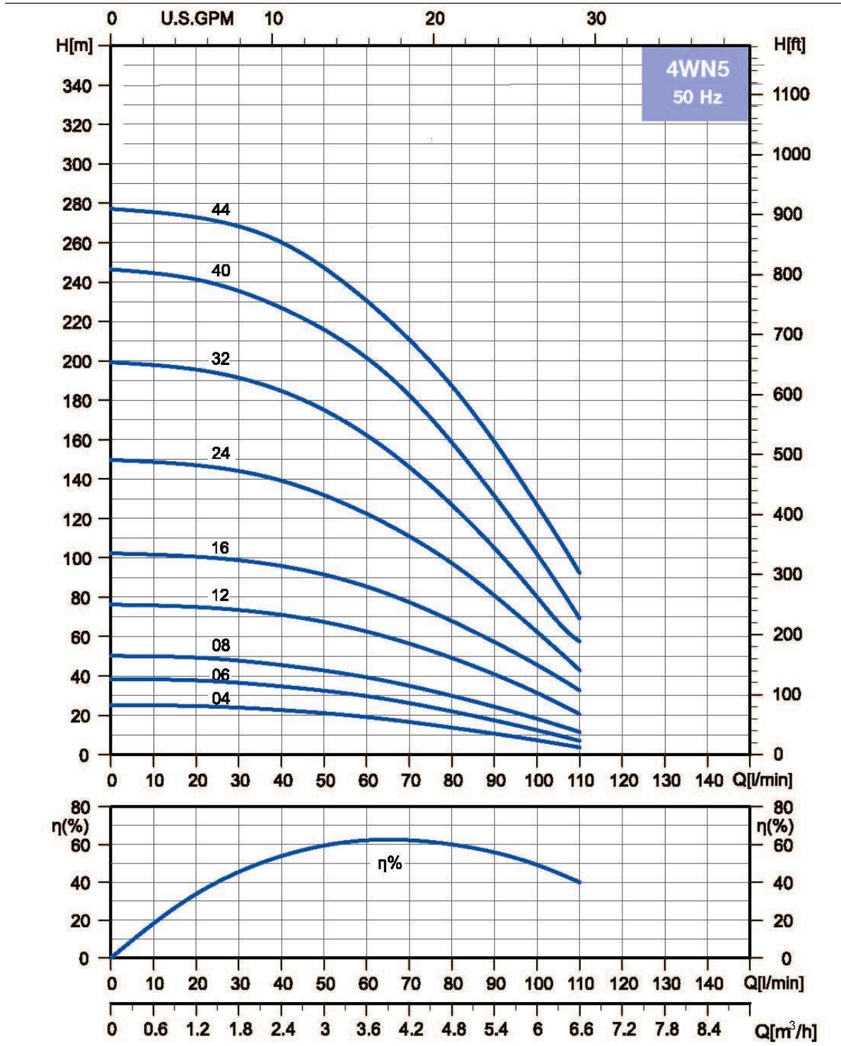
4WN5 – MEI > 0.60
